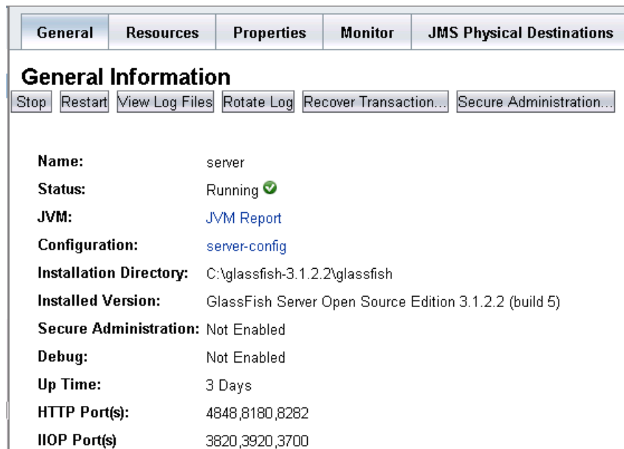
Рисунок 2. Окно свойств сервера
